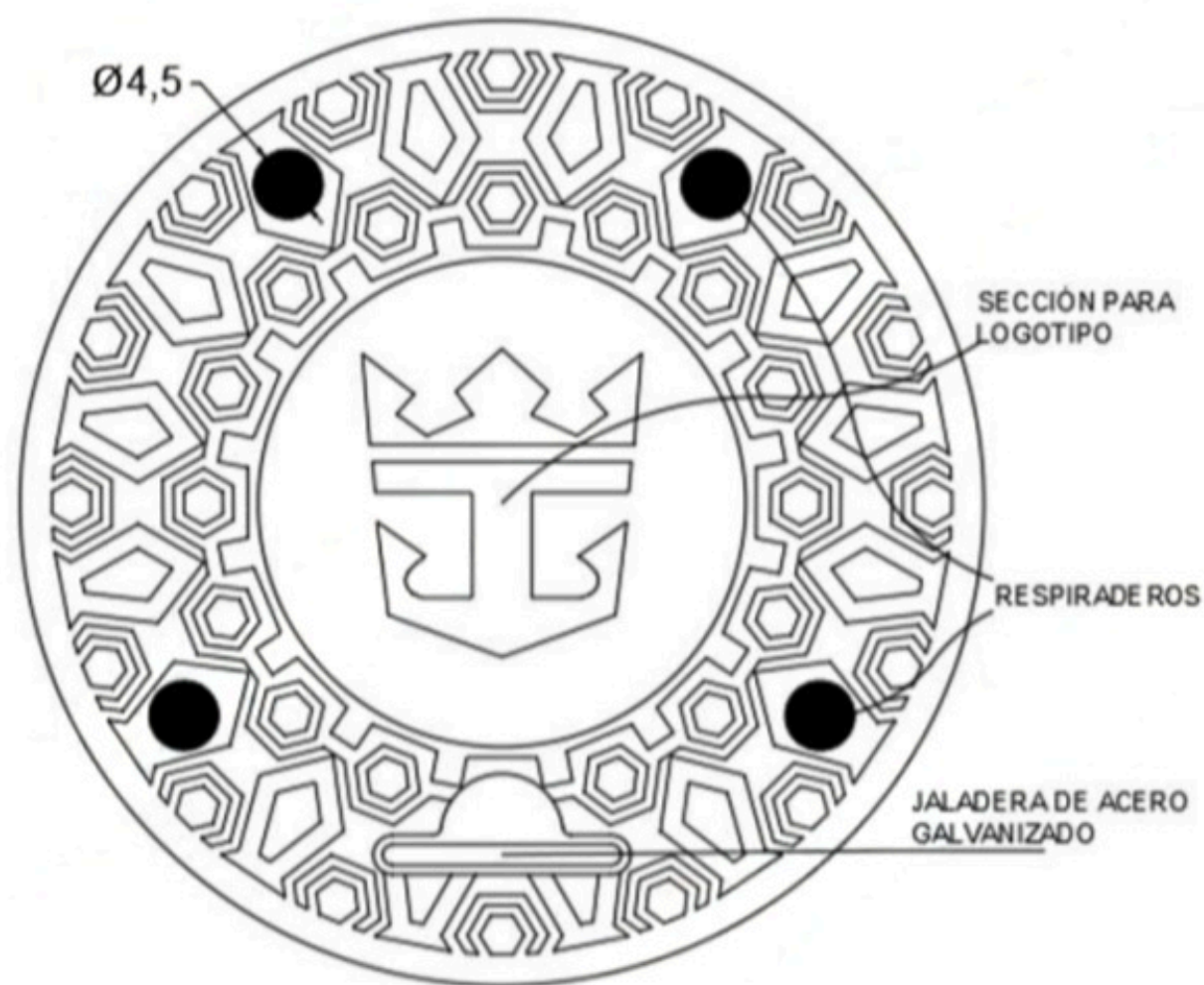
VISTA SUPERIOR
