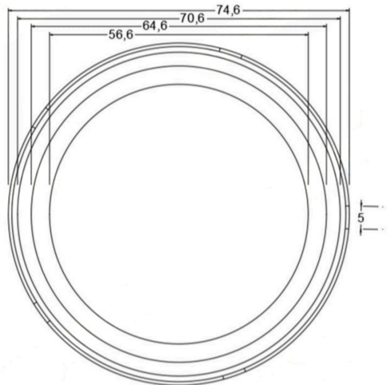
VISTA SUPERIOR
