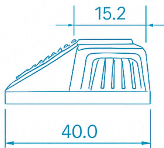
VISTA LATERAL
