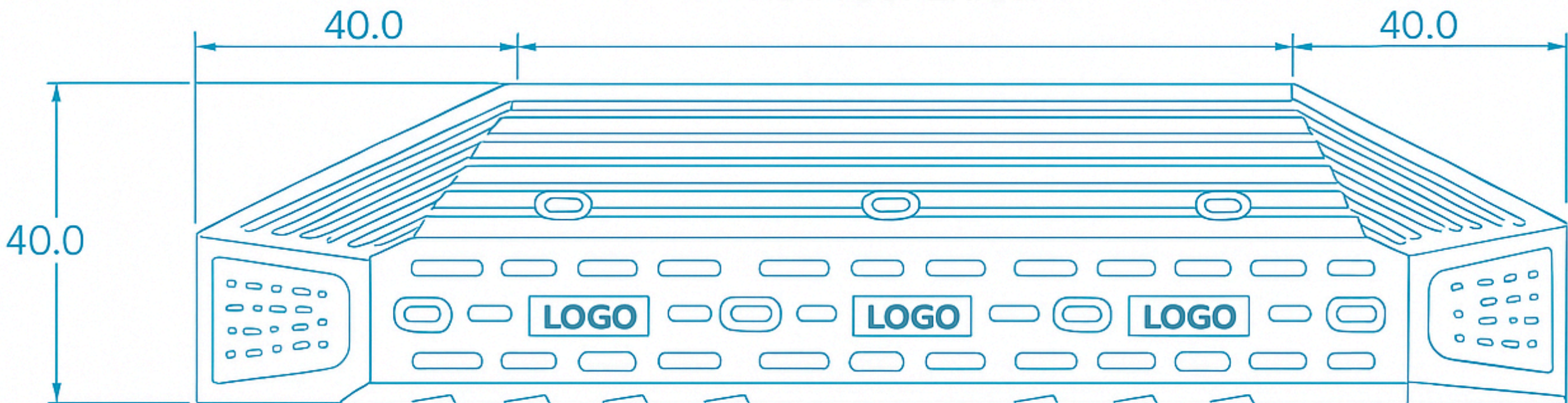
VISTA SUPERIOR
