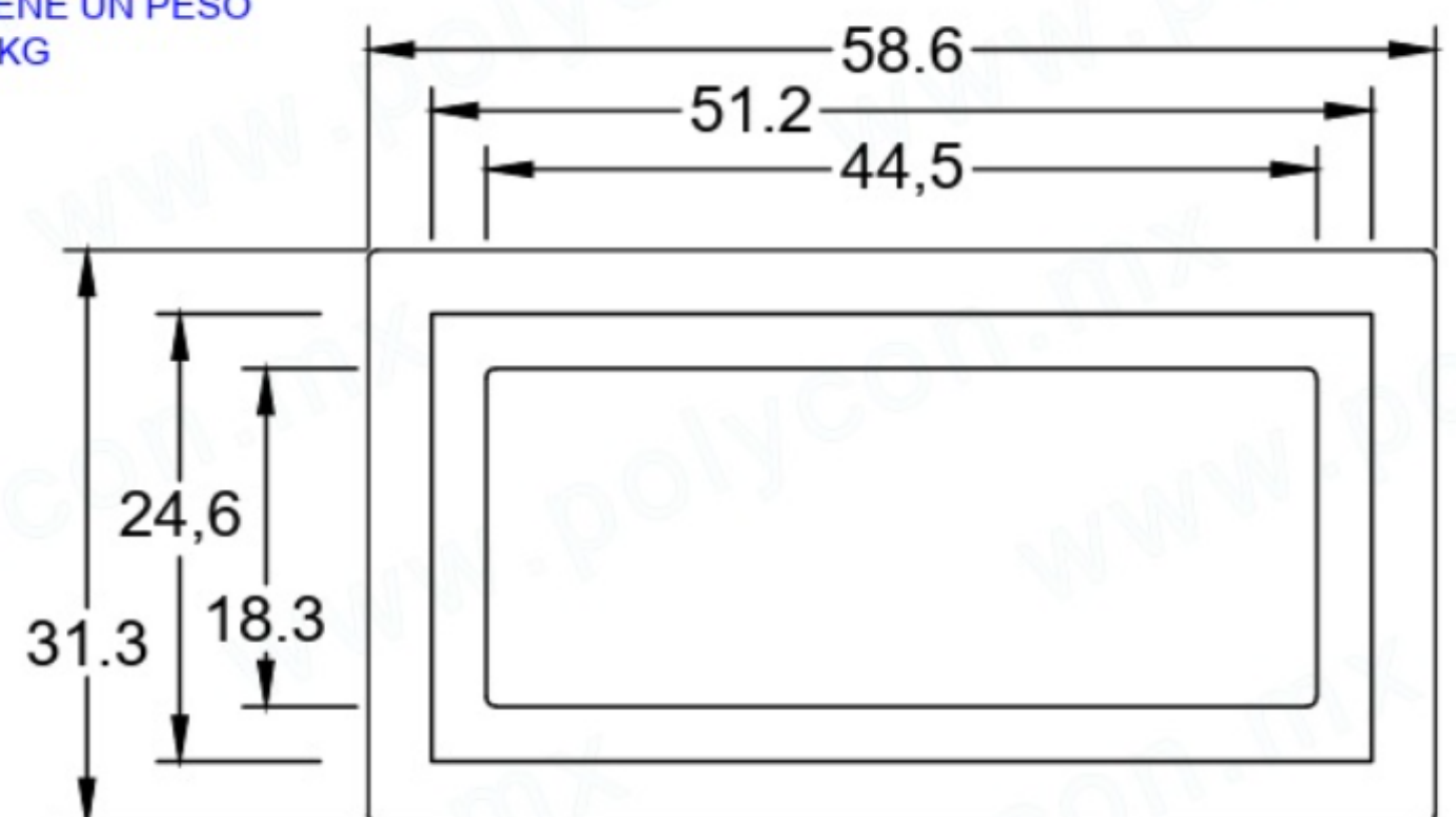
VISTA SUPERIOR
