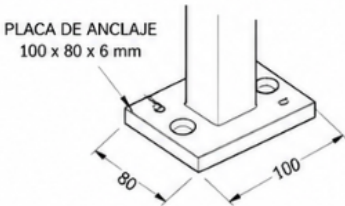
DETALLE ANCLAJE PATA ESCALA 1 : 2
