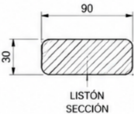
DETALLE LISTÓN ESCALA 1 : 2
