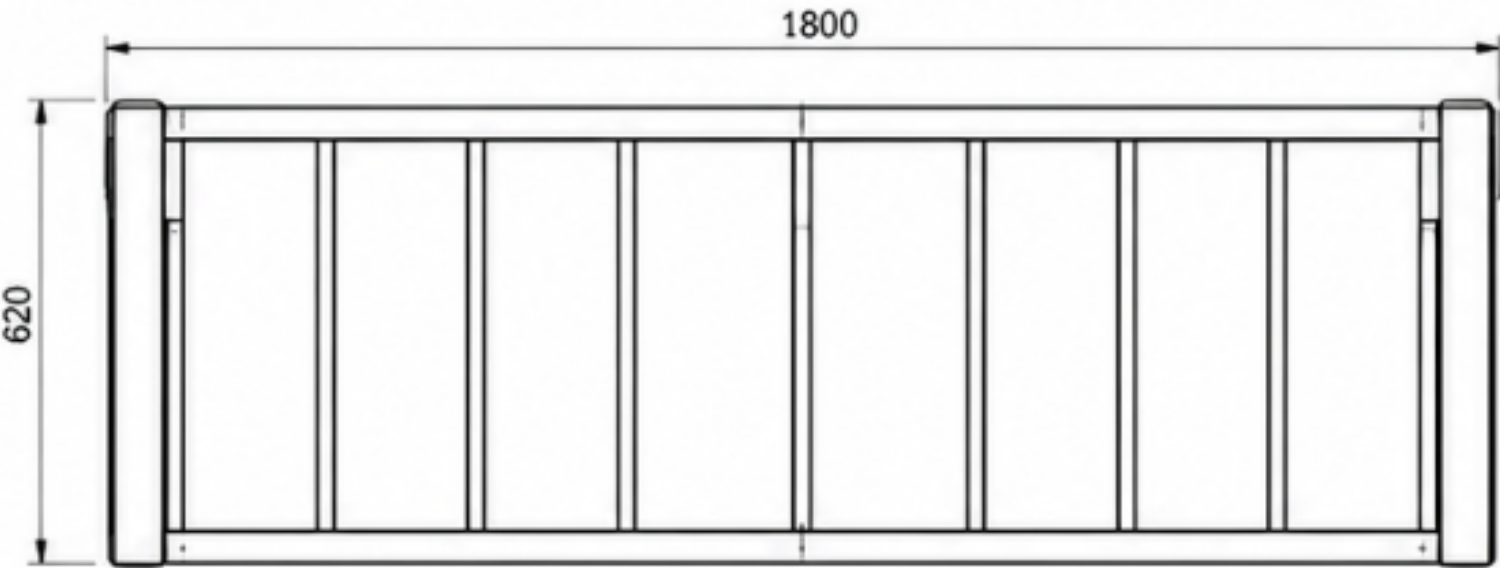
VISTA SUPERIOR
