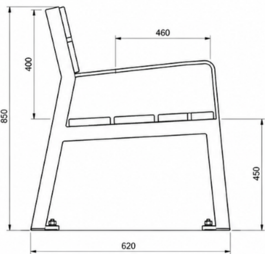
VISTA LATERAL
